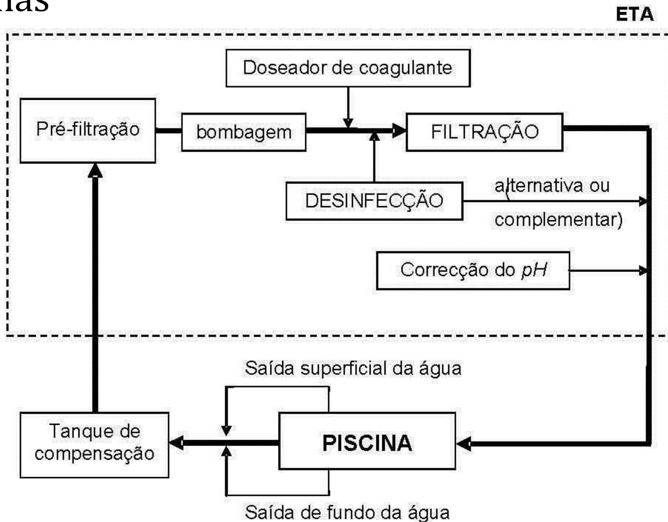
Figura 1 – Esquema de tratamento numa piscina típica
